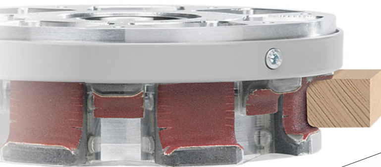
Uni-Line 7+7 kombiniertes Werkzeug aus 2 Schleifscheiben
