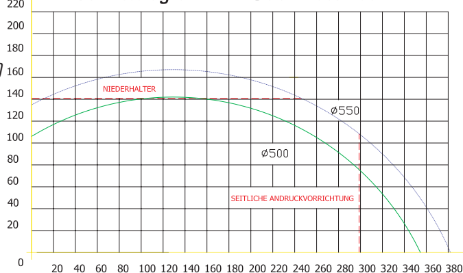
Schnittdiagramm KP 500 - Automat
