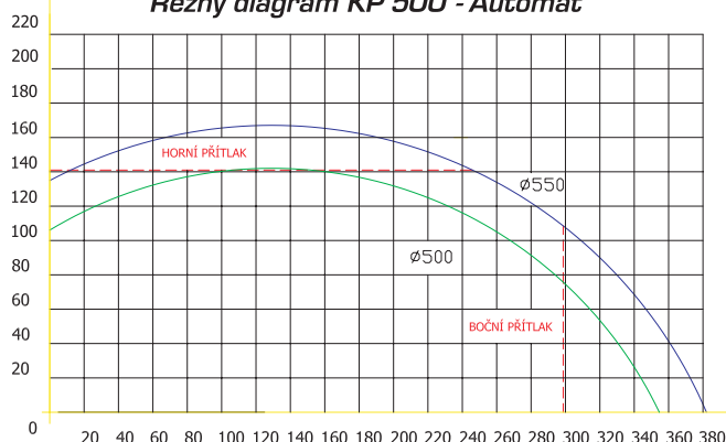
Řezný diagram KP 500 - Automat
