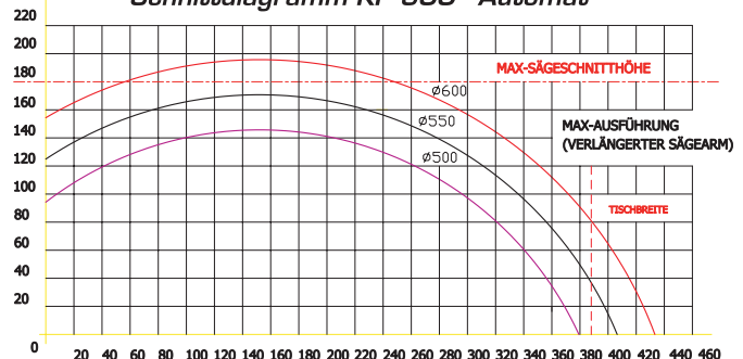
Schnittdiagramm KP 900 - Automat
