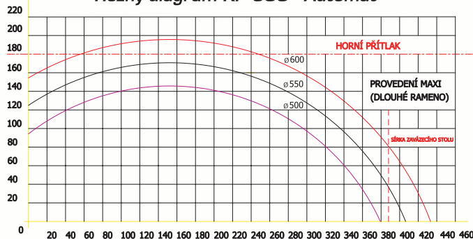
Řezný diagram KP 900 - Automat
