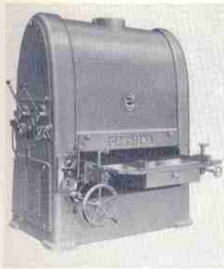
Fein- und Kontaktschliffautomat „FKA Junior 2“ mit 2 Bändern, jedoch 3 Schleifelementen
