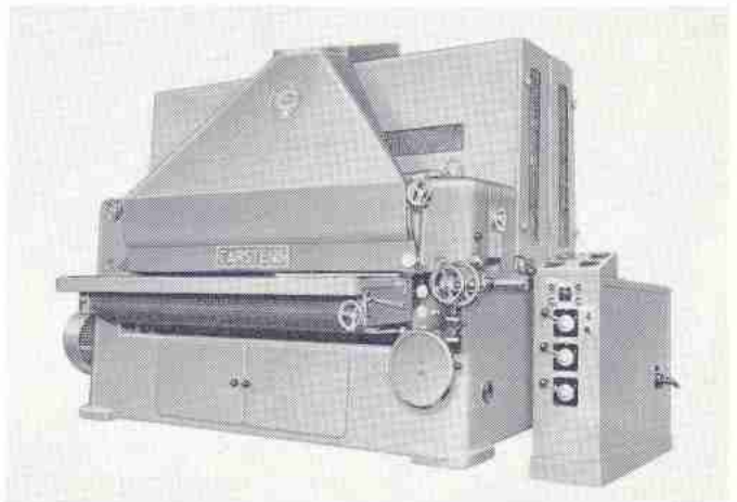
Kombinierte Großzylinder-Breitbandschleifmaschine „GZKK“ (1 Großzylinder und 2 Kontaktwalzen)
