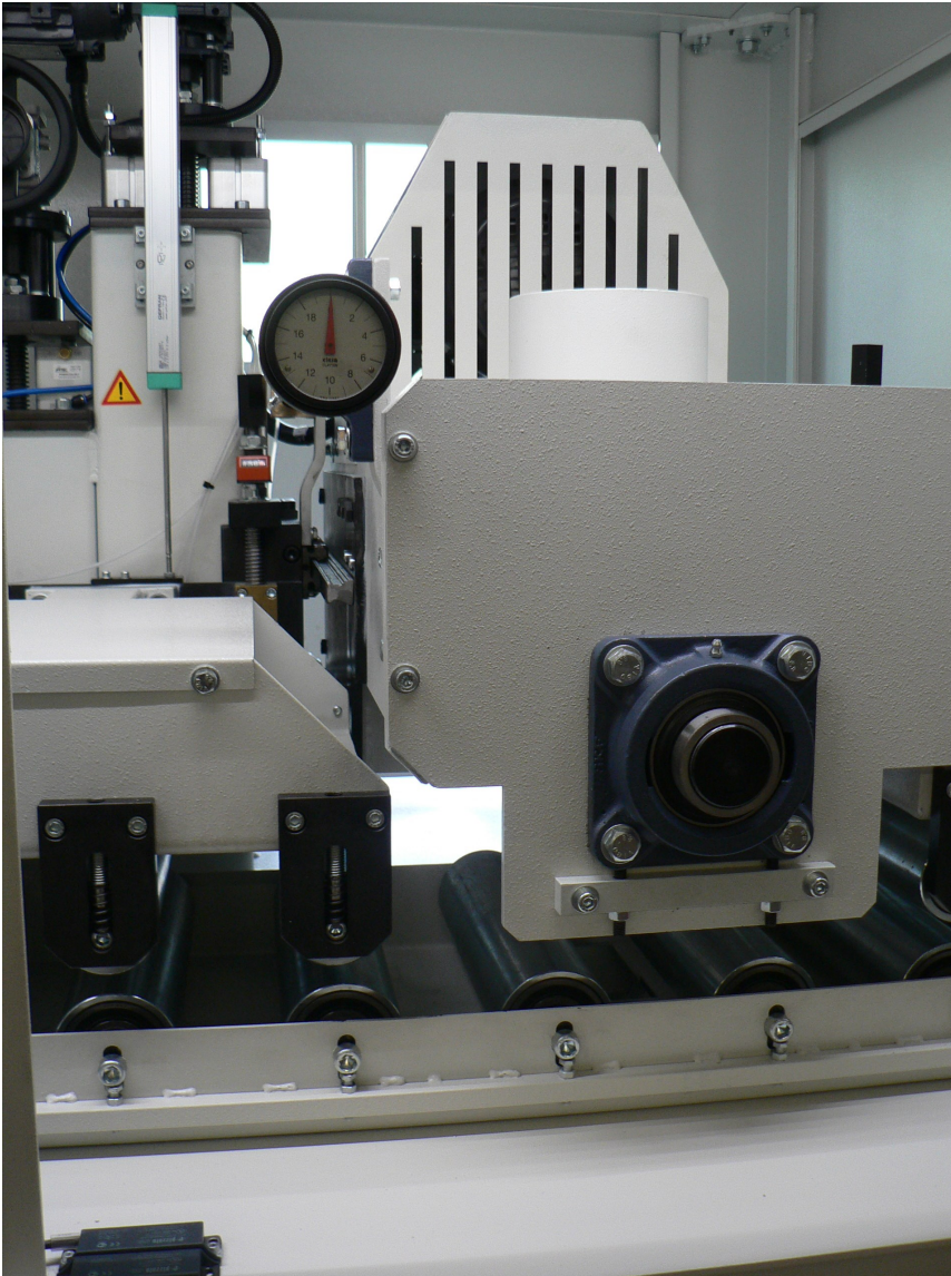
Starre Struktur der obere Arbeitseinheit
