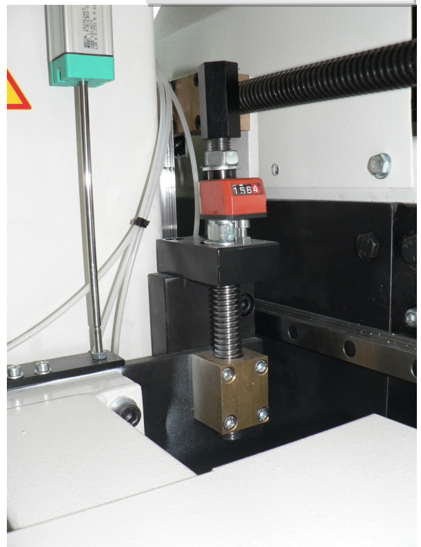
Verschiebungen durch Kugelumlaufführungen
