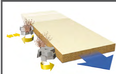
0,75+1,1 Kw 12.000 rpm
