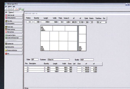
Visualizzazione in scala dello schema di taglio. Graphic display on scale of cutting patterns.
