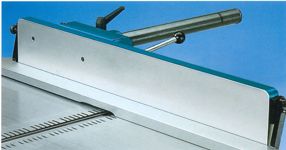
Guida supplementare mobile per lavorazione pezzi piccoli. Additional moving fence to work short pieces. Schwenkbarer Hilfsanschlag für Bearbeitung der kleinen Werkstücke. Guide supplémentaire mobile pour usinage des pieces petites. Guia extra mobile para el trabajo de piezas pequeña.
