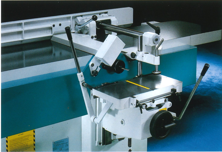
Gruppo cavatrice (a richiesta) Mortising attachment (on request) Langlochbohrereinrichtung (sur demande) Groupe mortaiseuse (auf anfrage) Dispositivo de taladrar (a pedido)
