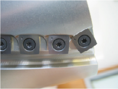
Planya kafa detayi
