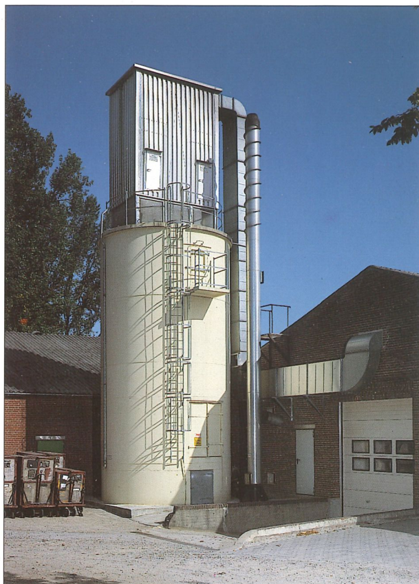
Deckenfilter, Typ PDF mit erhöhtem Einblasraum und Alutrapezverkleidung
