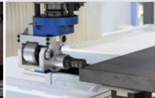
Чистовое фрезерование с ощупыванием свесов кромки на профиле постформинг
