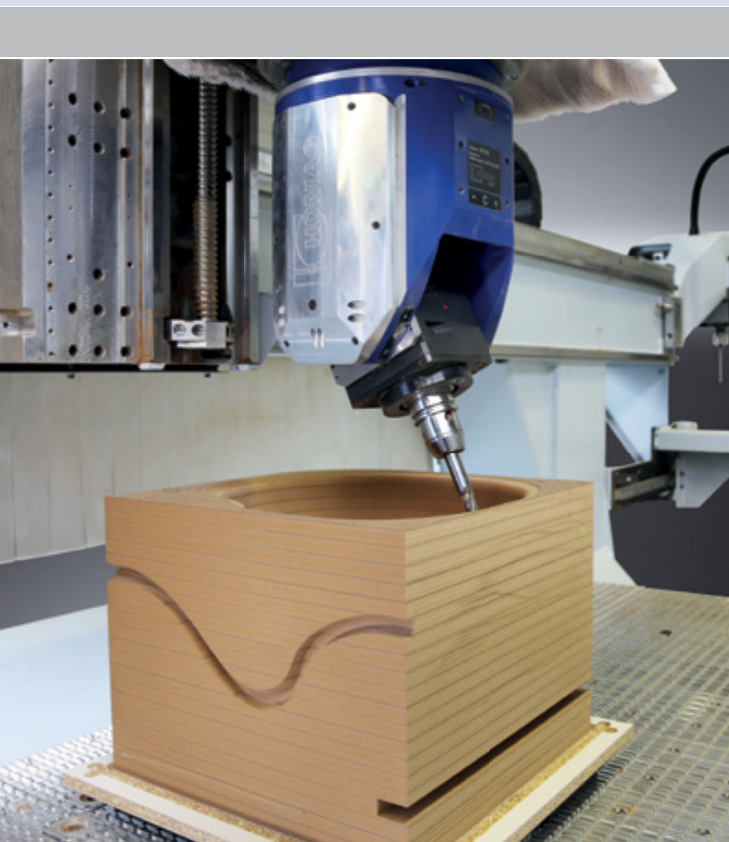
Фрезерная обработка конструктивных деталей с Z - высотой
