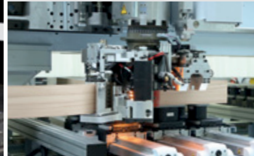
Облицовка кромки деталей до 100 мм высотой
