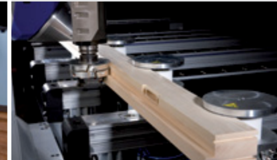
Профильная обработка деталей рам
