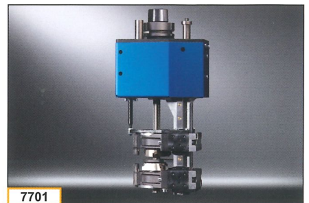
Bündigräsaggregat zum getasteten Profilieren von Werkstückkanten zeitgleich von oben und unten, z. B. Treppenstufen
