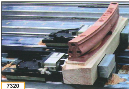
Klemmvorrichtung für Pfosten und Kanten
