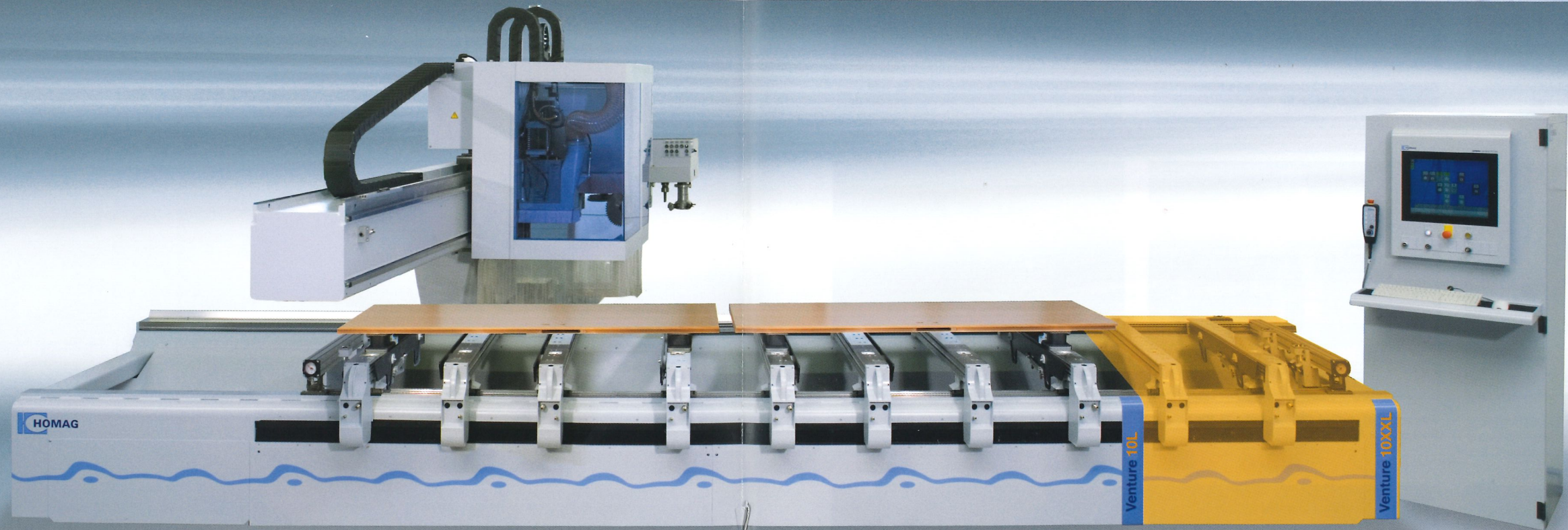
Flexibilität pur – Durch die integrierte FLEX5 Schnittstelle kann jederzeit die automatische Winklereinstellung nachgerüstet werden. Ein einzigartiges Feature zum präzisen Durchführen von Schiffschnitten oder Bohren und Fräsen in „jedem“ Winkel ohne manuelle Einstellungen
