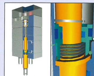
Automatische Spindelretrierung: patentiertes System für eine immer exakte Bohrtiefe bei unterschiedlichen Werkstoffen
