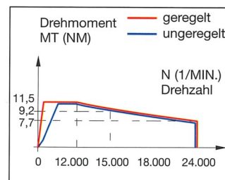
Hauptspindel (15 kW) mit geregelter Spindeldrehzahl 100-24.000 1/min. für ein extrem starkes Drehmoment auch bei geringen Drehzahlen wie z. B. beim Schleifen. Ein Spindelsensor sorgt für den Schutz der Hauptspindel bei z. B. Werkzeugunwucht
