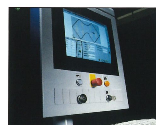
power control Steuerung PC 85: mit schwenkbarem Bedienpult für die einfache Maschinenbedienung durch Features wie Graphische Werkzeugdatenbank und Maschinendatenerfassung (MDE)
