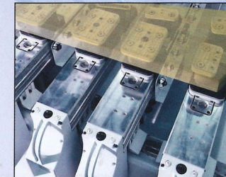
Arbeitstisch mit 8 oder 10 Konsolen und präzisen Linearführungen zur optimalen Werkstückspannung bei schwerer Zerspanung
