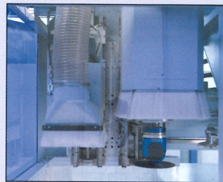
Zwei separate Z-Achsen für Hauptspindel und Bohrkopf ermöglichen den schnellen wechselnden Einsatz von Hauptspindel und Bohrkopf
