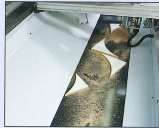
Hochsteifes Maschinenbett mit integrierter Reststück erfassung über die gesamte Bearbeitungstiefe von 1.600 mm. Es fallen keine Reststücke vor die Maschine (optional mit Späntransportband)
