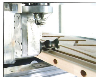
Interpolierende C-Achse 360°: Um die Aggregate in beliebigem Winkel drehen zu können, inkl. Druckluftübertragung in die Aggregate (z. B. zum Abblasen von Spanresten oder für getastete Bearbeitungen)
