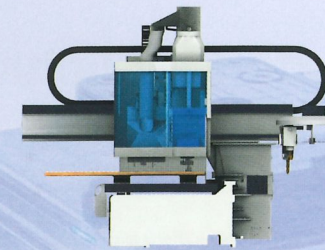
Aufgrund der kompakten, transparenten Sicherheitshaube können übergroße Werkstücke über das Maschinenbett hinaus stehen
