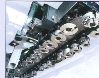
Schneller Kettenwechsler mit 30 großen Plätzen für Werkzeuge und Aggregate mit einem Durchmesser von bis zu 180 mm
