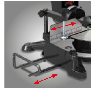
Verstellbare Anschlagschienen bei KGZ 255 E und KGZ 305 E sowie seitlich ausziehbare Auflagehilfen rechts und links
