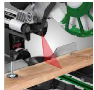
Laserprojektion auf das Werkstück zur genauen Kontrolle der Schnittposition
