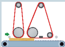
PRACOVNÍ JEDNOTKA RC DVA PRACOVNÍ VÁLCE + PEVNÁ MECHANICKY NASTAVITELNÁ PATKA
