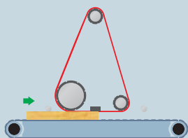
PRACOVNÍ JEDNOTKA TYP C PRACOVNÍ VÁLEC + PEVNÁ MECHANICKY NASTAVITELNÁ PATKA
