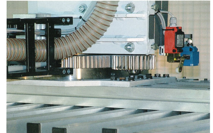
Drehvorrichtung des Portalroboters Turning device of the gantry robot
