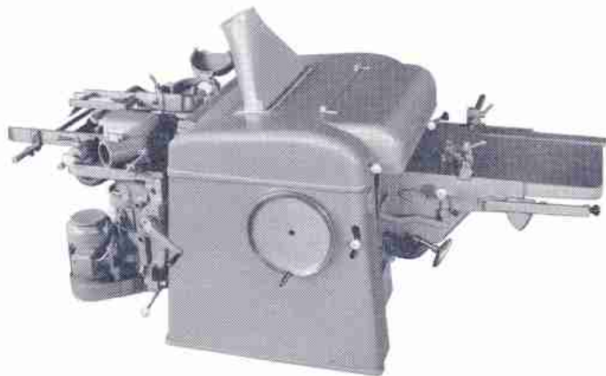
Ein-, zwei- und mehrseitige Tischhobelmaschinen, 500 und 630 mm Arbeitsbreite, auch mit zusätzlichen Arbeitswellen · Abgebildet ist Modell HTAF.
