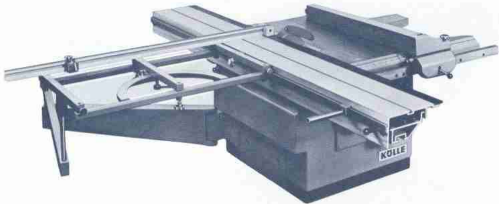
Format- und Besäumkreissäge KÖLLE KFS 4 380 V 7,5 bis 10 PS, wahlweise m. Vorritzmotor 3000/ 4000/ 5200 n der Sägenwelle, Schnitthöhe bis 135 mm, Besäumlänge 3000 mm, mit schrägstellbarem Kreissägeblatt, 600 kg
