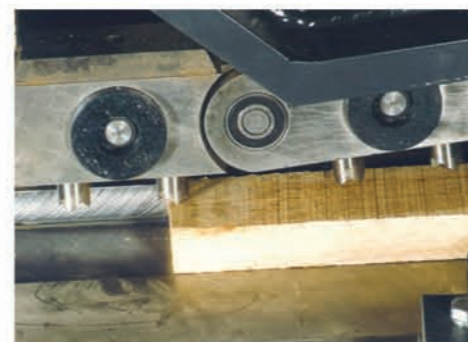
Uzdužno profiliranje Longitudinal profiling
