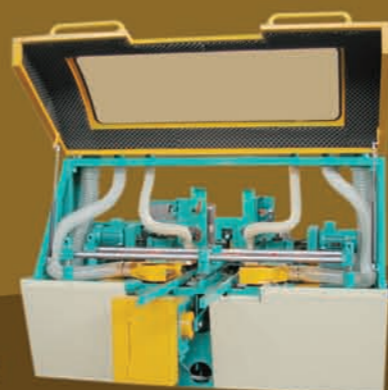
Uzduno profiliranje Longitudinal profiling
