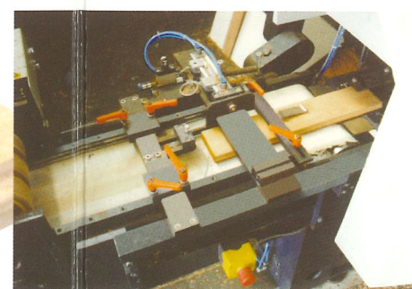
Автоматическая загрузка Vending device
