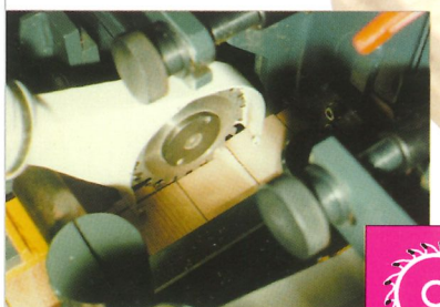
Подрезатель Pre-cutter
