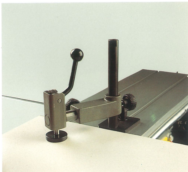
8.2.2. APRETADOR MANUAL ECCENTRIC HAND CLAMP PRESSEUR MANUEL EXZENTER-SPANNVORRICHTUNG
