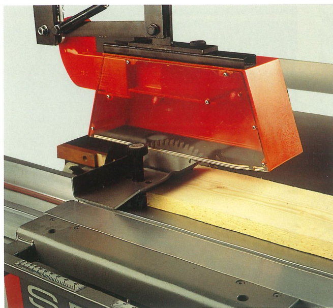
8.10.2 TOPE SOBRE CARRO CLAMPING SHOE BUTÉE SUR LE CHARIOT KLEMMSCHUH AUF WAGEN
