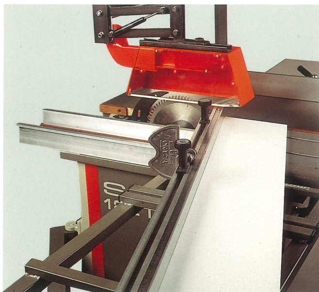
INGLETE MITRE FENCE GUIDE D'ONGLET GEHRUNGSANSCHLAG
