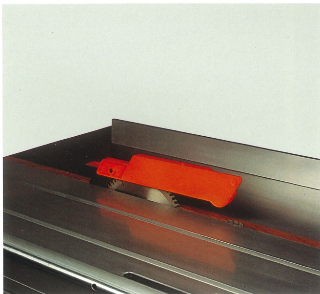
PROTECTOR STANDARD SAFETY HOOD CAPOT PROTECTEUR SCHUTZHAUBE
