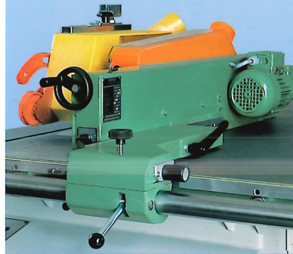
Verstellung mit Kreissägenanschlag
