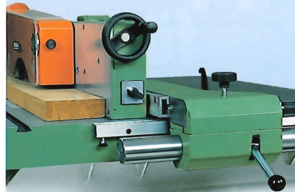
Befestigung am Kreissägenanschlag
