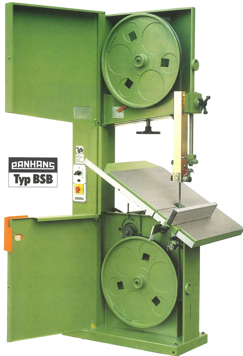
Mechanische Höhenverstellung der oberen Führung durch Handrad und Sperritzel. Kontrollfenster für den Blattlauf.
