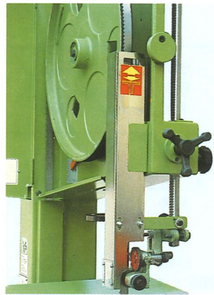
Mechanische Höhenverstellung der oberen Führung durch Handrad und Sperritzel. Kontrollfenster für den Blattlauf.
