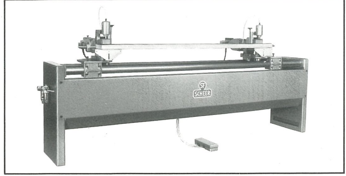
DB 10/2200 mit 2 parallel zueinander stehenden Bohraggregaten
