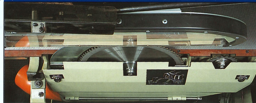
Tür zum Sägeblattwechsel mit Schnellverschlüssen und Mikroschalter.
