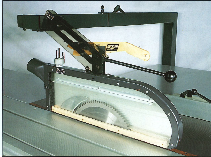
Parallelogramm-Schutzhaube mit 80 mm Absaugstutzen und Höhenansläge je nach Sägeblattdurchmesser.
