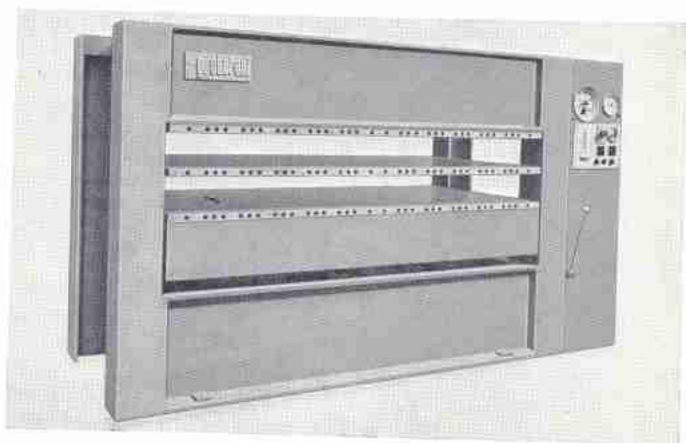
Hydraulische Presse Typ PA/240 mit 240 t Gesamtdruck und gebohrten Stahlheizplatten
