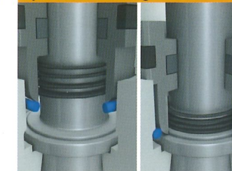
Automatische Spindelklemmung
