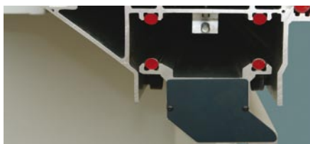
Podwójnie ułożyskowany stół formatowy.
