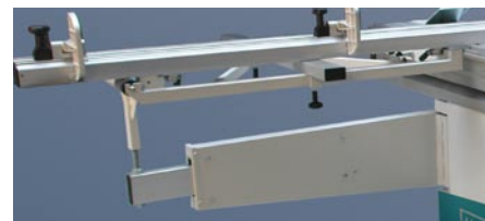
Przykładnica kątowna rozciągnięta do 3250 mm.
