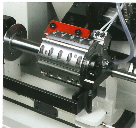
Riaffilatura automatica dei coltelli da pialla nella testa portacoltelli con bloccaggio tradizionale o idraulico
