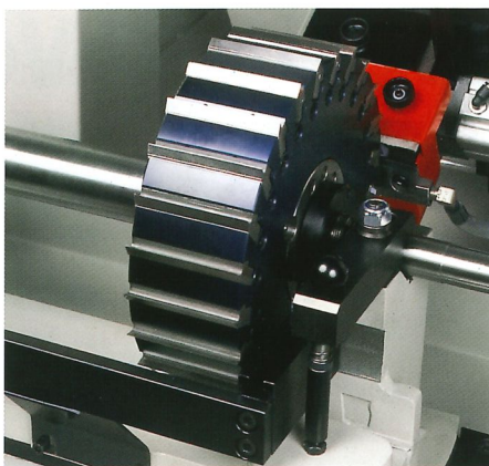
Divisore automatico per fino a 36 taglienti
