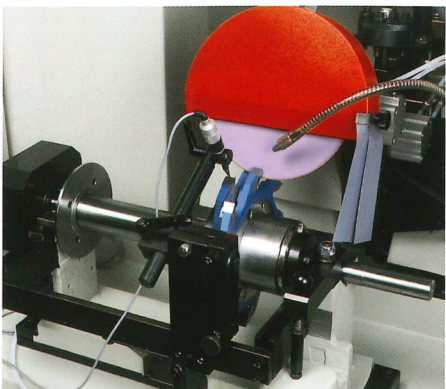
Riaffilatura automatica delle frese
