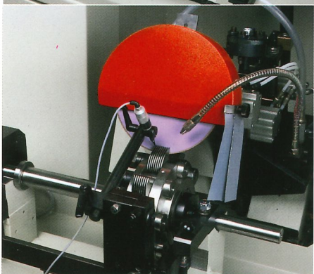
Riaffilatura automatica di utensili per giunzioni a pettine. Dispositivo integrato per l'allineamento delle frese per giunzioni a pettine.
