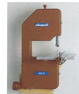
Bandsäge-Einrichtung
