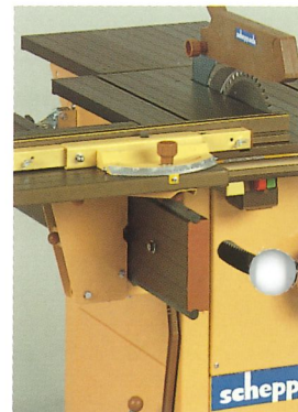
Schiebeschlitten
