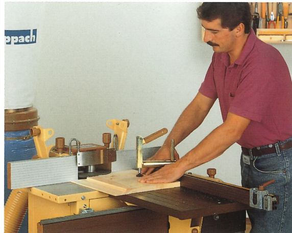
hf 3000 mit Schiebeschlitten
