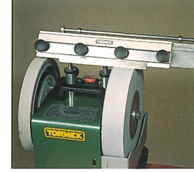
Schleifvorrichtung SVH-320 für Maschinenhobelmesser
