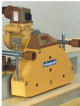
Vorschubapparat
