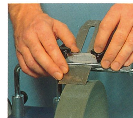
Schleifvorrichtung SVH-60 für Hobeisen
