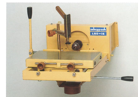
Langlochbohr-Einrichtung
