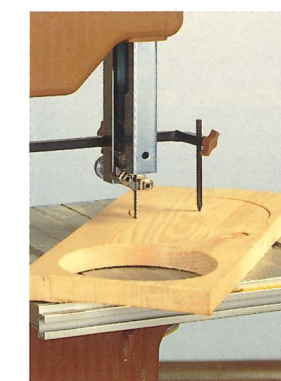
Kreisschneid-Einrichtung
