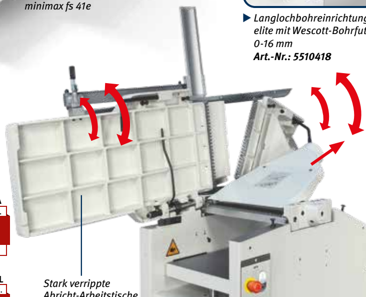
minimax fs 41e mit geöffneten Abrichttischen
