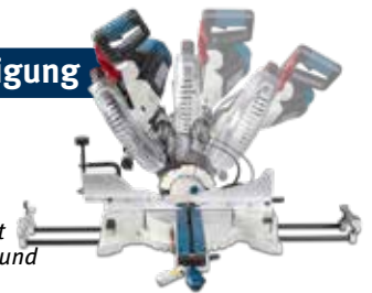
Ausziehbare Anschlagsschienen und ausziehbarer Tisch
