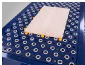
Steckbare Anschläge zur Fixierung des Werkstücks
