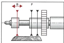
Einschnittmöglichkeiten mit Blattverstellung bis zu 6 Blättern Cutting options for movable cutter heads up to 6 movable blades
