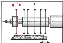
Possibilités de coupe avec lames de scie mobiles jusqu'à 6 lames mobiles
