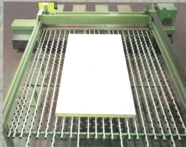
Mikro-Einschübe für den paketweisen Einschub dünner Platten Micro-infeeds for feeding thin and wavy panels Micro-alimentateurs pour l'alimentation de panneaux minces en paquets Micro-alimentadores para la alimentación de paquetes de tableros delgados Micro-introduttori per l'introduzione di pannelli sottili a pacco
