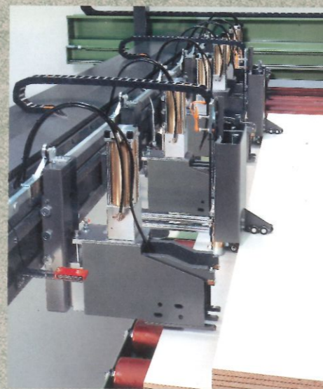
Beschickung eines Plattenpaketes Infeed of book of panels Alimentation d'un paquet de panneaux Alimentación de paquetes de tableros Carico di un pacco di pannelli
