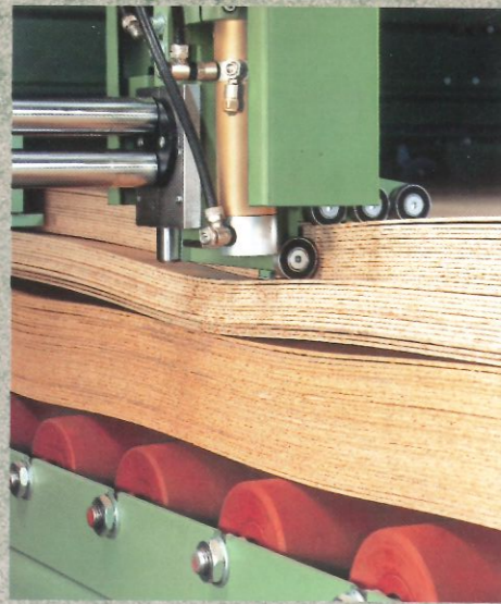
Mikro-Einschübe für den paketweisen Einschub dünner Platten Micro-infeeds for feeding thin and wavy panels Micro-alimentateurs pour l'alimentation de panneaux minces en paquets Micro-alimentadores para la alimentación de paquetes de tableros delgados Micro-introduttori per l'introduzione di pannelli sottili a pacco
