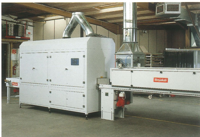
UV-Kanal mit vorgeschalteter IR- Abluftzone
