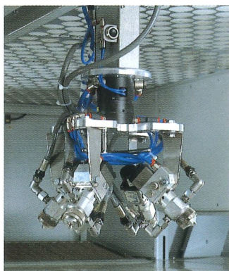
Pistolen-Schnellwechsler
