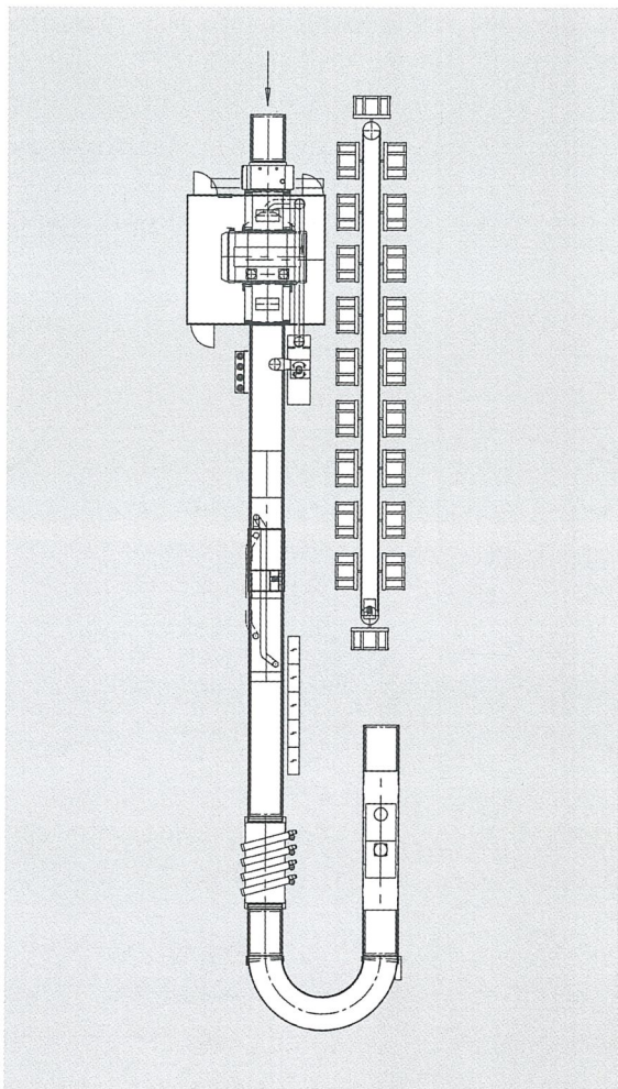
Lackieranlage für Wasser- und Lösemittel-Lacke mit Kälte- und UV-Trockner Finishing line for water and solvent based lacquers with cold air- and UV-dryer
