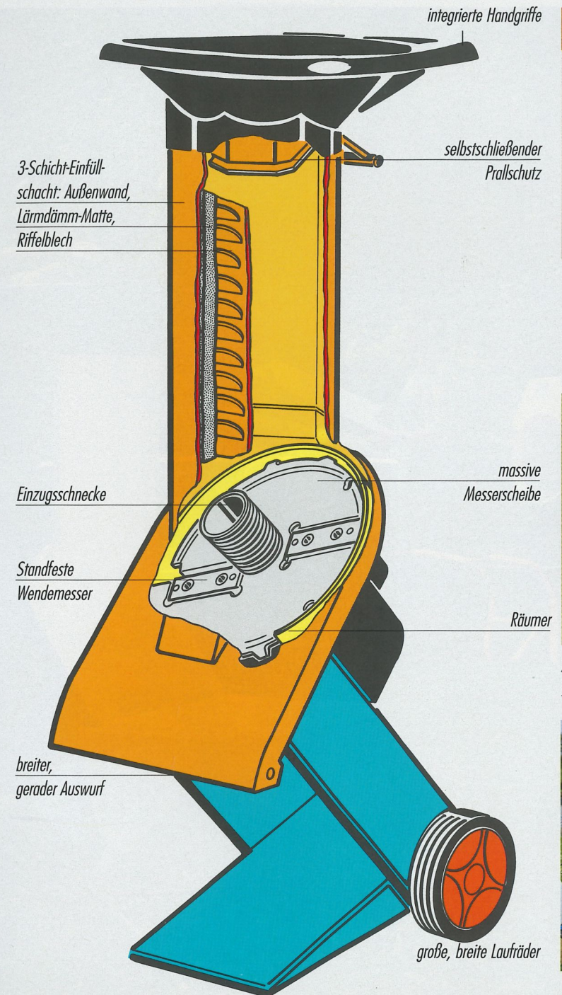
Die Häckselmesser aus Spezialstahl bleiben lange scharf. Es sind Wendemesser, die im Bedarfsfall im Handumdrehen gewendet oder ausgetauscht werden können. Sie sind auch nachschleifbar.
