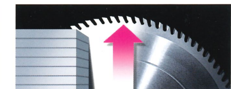
Automatische Überstandregulierung , entsprechend den Pakethöhen, um auch bei wechselnden Schnitthöhen eine optimale Schnittqualität sicherzustellen.
