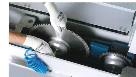
Hauptsäge- und Vorritzerggruppe mit Schnellspannsystem für die Werkzeuge. Chariot de la scie avec déblocage rapide de la lame.
