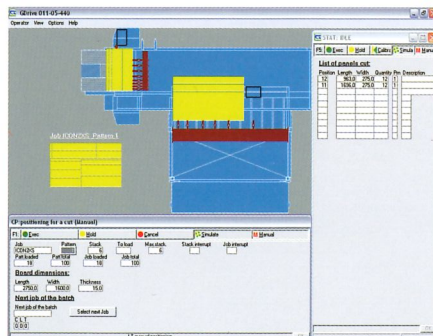
Grafische Echtzeitsimulation der Ausführungsphasen (RTG System).
