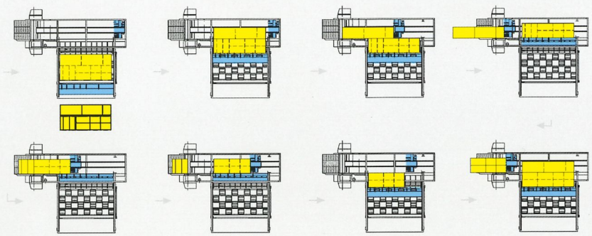
Schnittplan mit Kopfschnitt in zweiter Phase für Platten mit einer Breite grösser als 1550mm Schéma avec coupe de tête en deuxième phase pour panneaux qui peuvent être plus large que 1550mm
