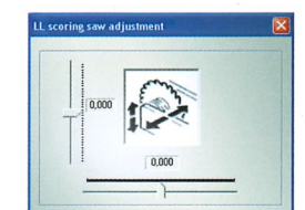
Elektrische Vorritzereinstellung vertikal und horizontal direkt über die Maschinensteuerung G-Drive.
