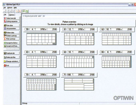
GIBEN OPTIWIN (optional auf Anfrage). Optimierungsoftware zur automatischen Erstellung von Schnittplänen unter Berücksichtigung des Verschnitts, der Zuschnittskosten und den effektiven Kosten für das zuzuschneidende Material.
