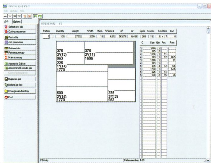
Masstabliche Anzeige des Schnittplanes (T-CUT Concept).
