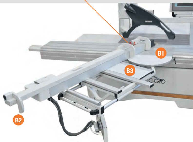
CARRO INCLINABILE +47° -47° CHARIOT INCLINABLE +47° -47° CARRO ESCUADRADOR INCLINABLE +47° -47°
