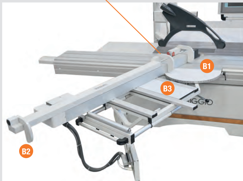
CARRO INCLINABILE +47° -47° CHARIOT INCLINABLE +47° -47° CARRO ESCUADRADOR INCLINABLE +47° -47°
