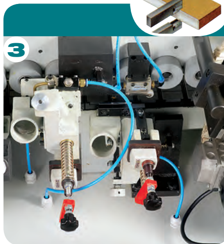
GRUPPO RASCHIATORE con lettore digitale numerico.
