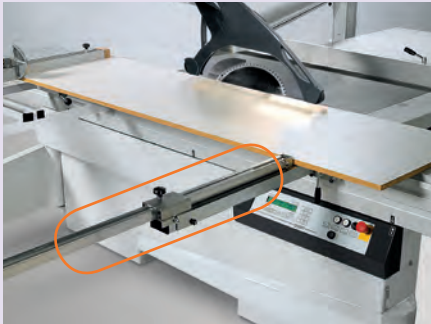
Option Pianetto tagli paralleli Tablette pour coupes parallèles Mesa para cortes paralelos
