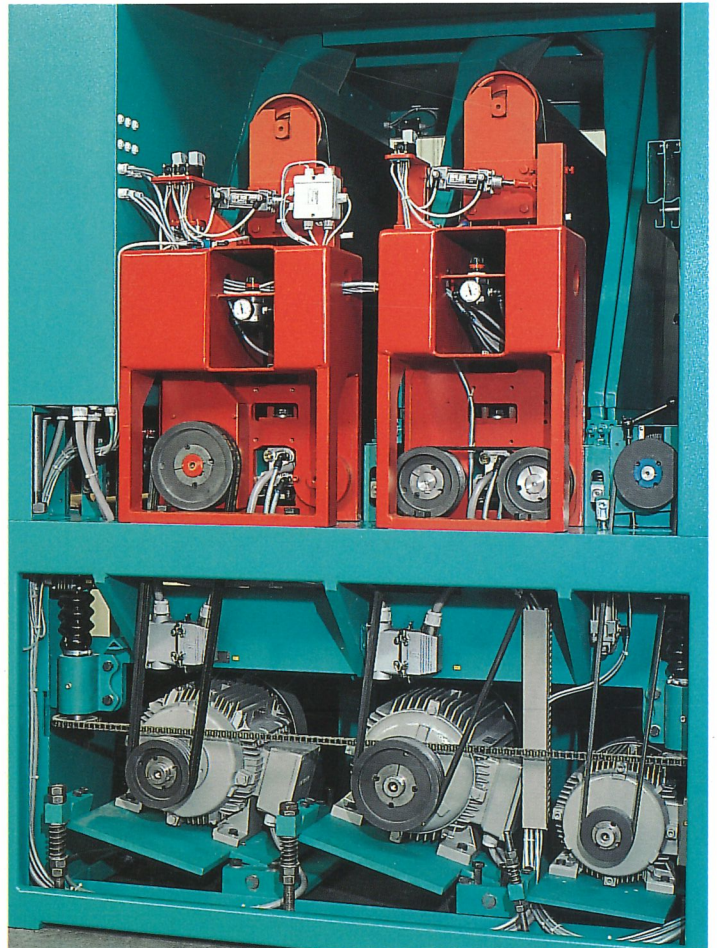
Schleifbandantriebsseite, technische optimale Kraftübertragung, alle zu wartenden Elemente sind übersichtlich und leicht zugänglich. Gut sichtbar die umlaufende Kette für parallele Tischhöhenverstellung und der Keilriemen mit Spannvorrichtung zum Antrieb der Reinigungsbürste. Die Antriebsmotoren sind jeweils auf einer einseitig drehbaren Konsole montiert, somit ist ein schnelles und leichtes Spannen oder Austauschen der Keilriemen möglich.
