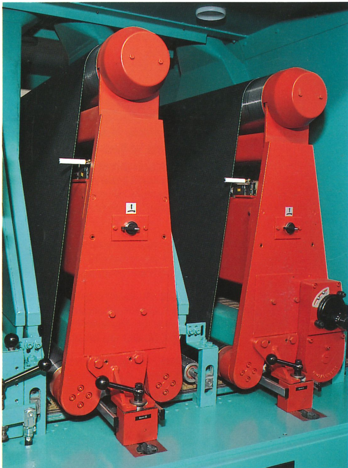
Die Schleifaggregate der Vega 2 C-E mit Combi-Aggregat und Schleifschuh. Sekundenschneller Wechsel und Spannen der Schleifbänder. Durch die automatische Zustellung der Schleifelemente ist die Bedienung denkbar einfach. Fehlbedienung durch Betriebsbereitschaftsanzeige ausgeschlossen. Gut sichtbar der 4-fach einstellbare Schleifbandkörnungsausgleich für die Kalibrierwalze.
