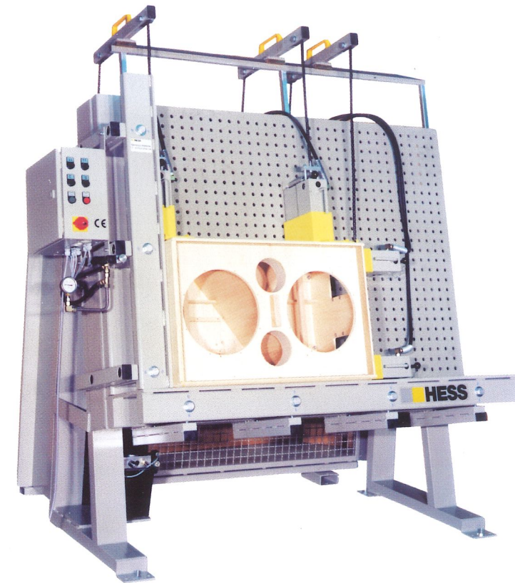
Hess-Sonderpresse, elektrohydraulisch. 1-stationig (auf Basis der Tischpresse). Arbeitsbereich: 1450 x 450 mm. Anschlaghöhe: 400 mm. Zum Ver- pressen von Lautsprecher-Boxen.
