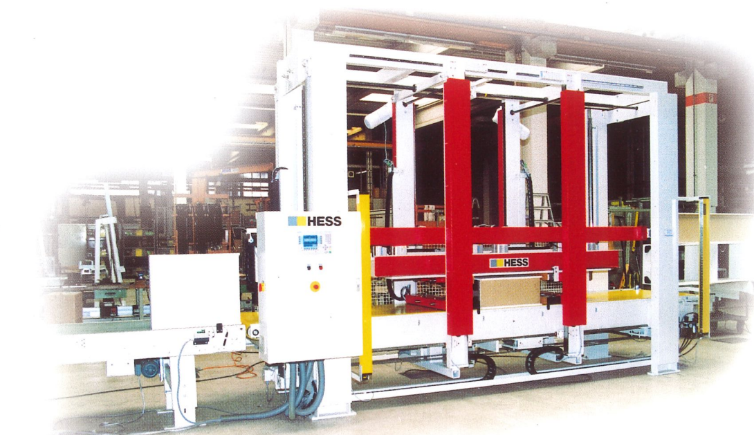
Hess-Formatic-linear-Druchlauf- presse. Maßabfragung über gespeicherte Datensätze oder mit Datenverbund Online. Schwere Bauweise.
