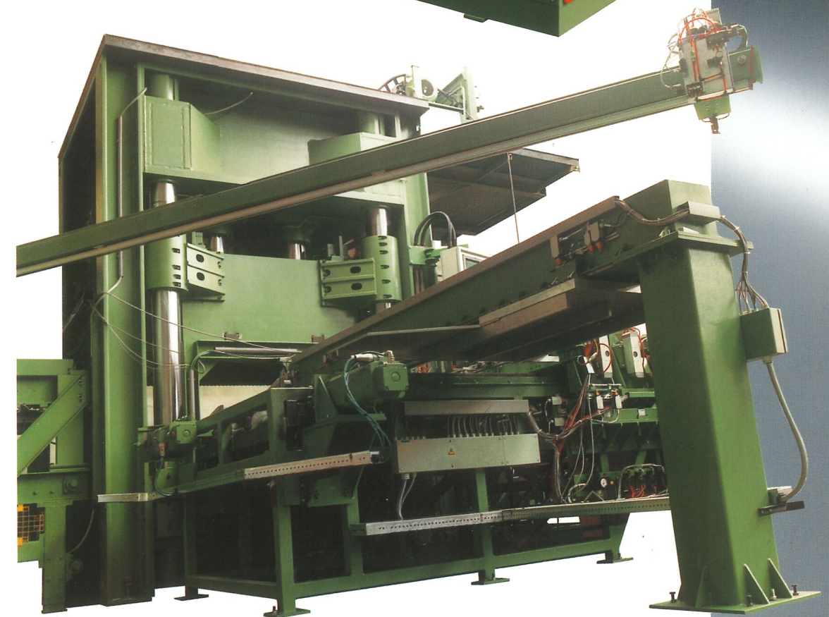
Trittrostpresse 700 to
