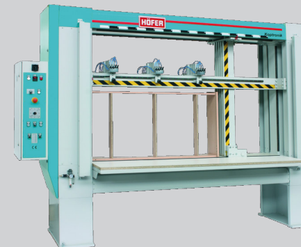
Korpuspresse - KOPTRONIK - Sonderausführung Case clamp KOPTRONIK - customized
