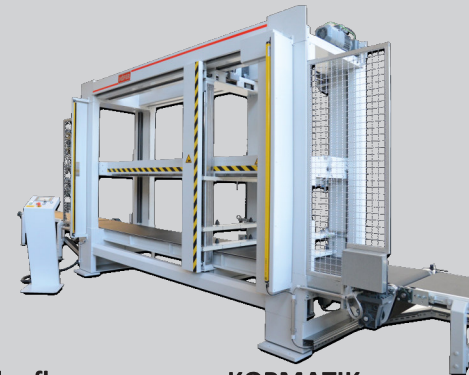
Durchlaufkorpuspresse - KOPMATIK Feed-through case clamp - KOPMATIK
