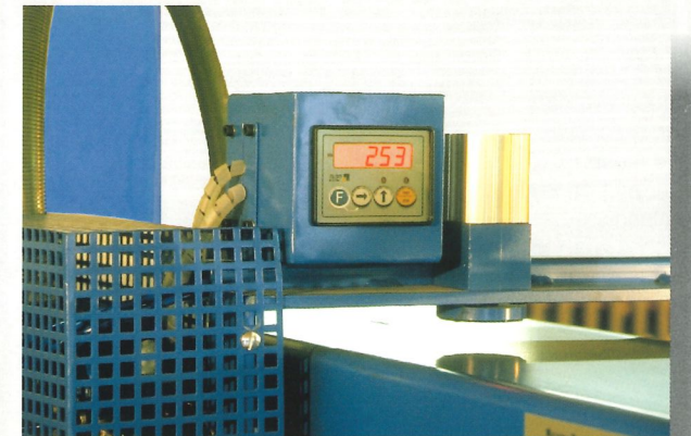
Affichage digital de l'angle des marches dans le limon Digital display of the stair position in the string Digitale hoek instelling voor de treden in de trapboom Winkeleinstellung mit digitaler Anzeige
