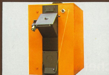
Spezial-Späne/Stückholzkessel für den Handwerksbetrieb
