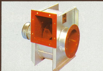
Rauchgasventilator
