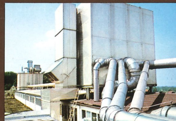
Filterhaus als Zwischenabscheider in einem Möbelwerk
