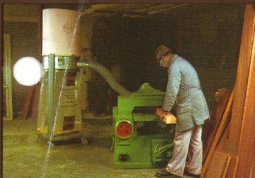
Fahrbare Absauganlagen
