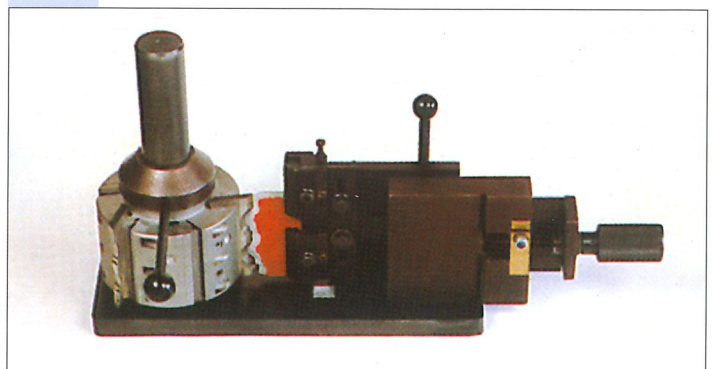
Jointervoreinstellgerät
