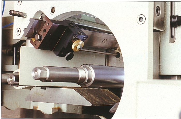
Fernbedienbarer Geradjointer mit automatischer Zustellung des Jointsteins. • Sicherheit! Auch bedienbar, wenn die Sicherheitsabdeckung geschlossen ist • Entfernt Scharten von den Geradmessern • Gewährleistet parallele Messer über die volle Arbeitsbreite
