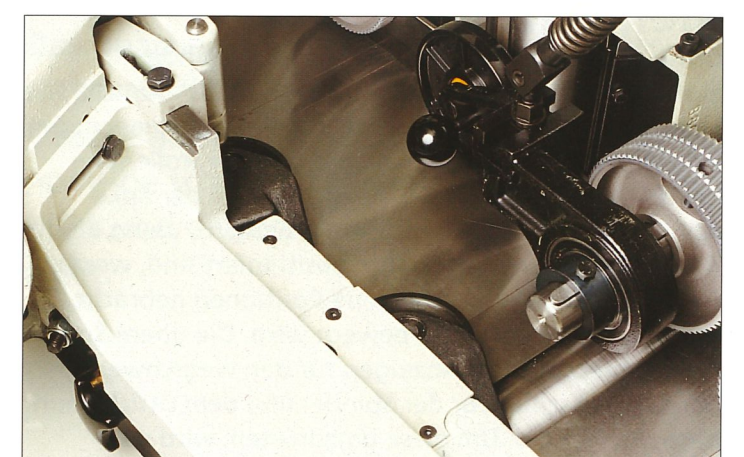
Seitliche Andruckrollen führen das Werkstück am rechten Anschlag. • Maximale Kontrolle von kurzen und schmalen Werkstücken, um eine bessere Genauigkeit und Oberflächenqualität zu erhalten
