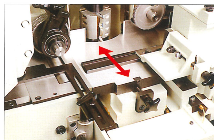
Tischplatten lassen sich im Bereich der Vertikalspindeln schnell auf den Flugkreis einstellen. • Maximale Auflage des Materials beim Profilieren • Reduzierte Umrüstzeit
