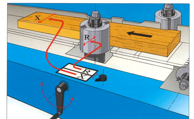
Weinig DigiSet erlaubt dem Bediener, den Werkzeugradius einzugeben und die Spindel auf das gewünschte Werkstückfertigmaß in Dicke und Breite einzustellen. • Schnelles Umrüsten der linken und oberen Spindel für Profilierung und Hobeln • Das erste Werkstück entspricht dem gewünschten Fertigmaß
