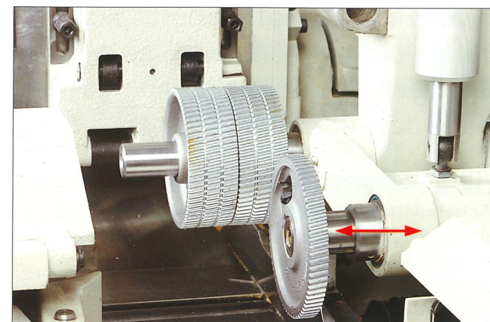
Axialverstellung der Vorschubwalze gegenüber der linken Spindel. • Schnelle Verstellung für breites und schmales Material • Eliminiert das zeitraubende Verschrauben von Vorschubwalzen
