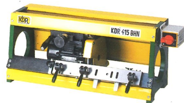
Tischmaschine für Scharfschleifen von Hobelmessern KDR 415 BHN, KDR 615 BHN Länge des Scharfgeschliffenen Messers 410 (610) mm
