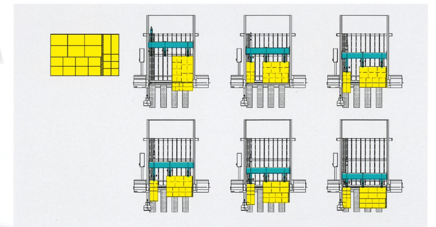
Queraufteilung der Kopfschnittportion GLEICHZEITIG mit der Längsaufteilung der Hauptportion.
