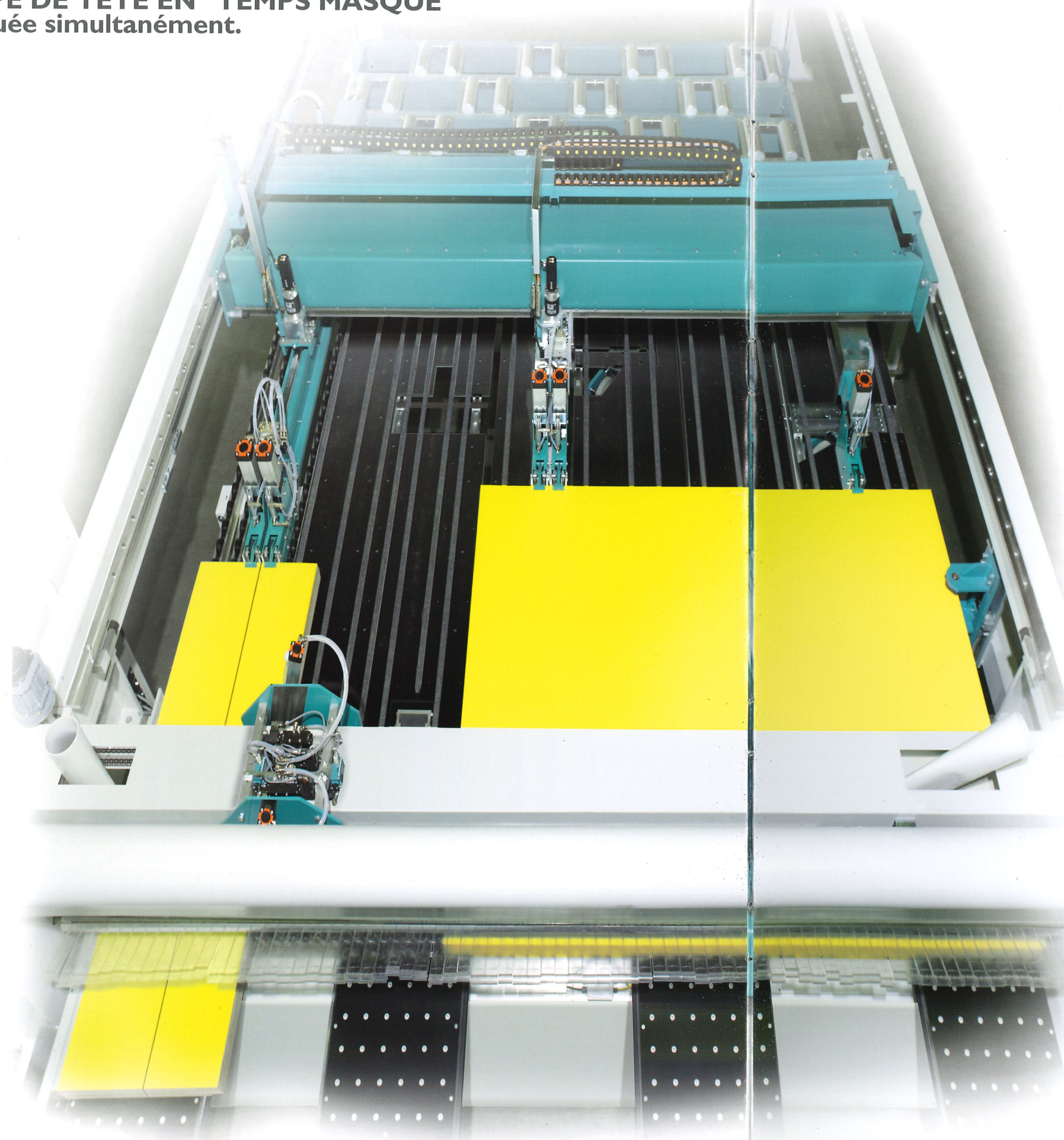
Queraufteilung der Kopfschnittportion GLEICHZEITIG mit der Längsaufteilung der Hauptportion.
