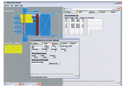
Grafische Simulation in Echtzeit der verschiedenen Bearbeitungsphasen.
