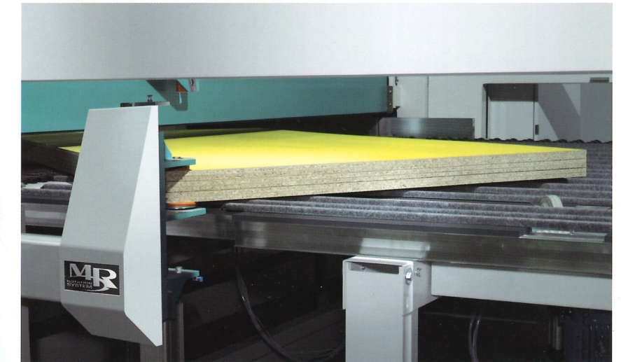
Spannzange "MR" für die Drehung der Plattenpakete.
