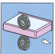
Schwabbelaggregat oben und unten mit Oszillation Zum Griffigmachen der Kanten mit Ausnutzung der gesamten Scheibenbreite.
